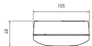
Met opbouwdoos (accessoire)
