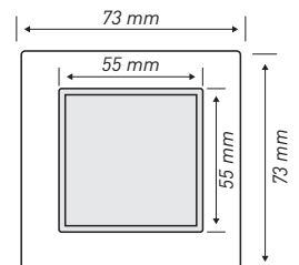
Met opbouwdoos (accessoire)
