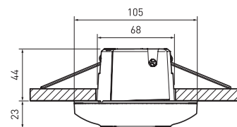
Met Flush mount spring clips (inbegrepen)
